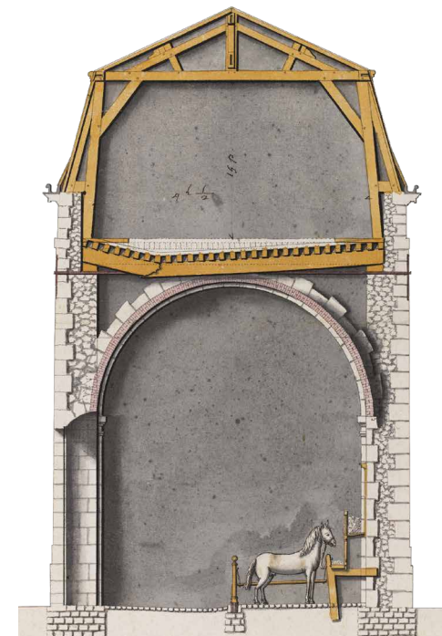
Profil de la Grande Écurie du Roi à Versailles, en 1695
